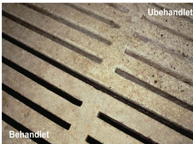
Spaltegulv efter ca. 2 års brug.
